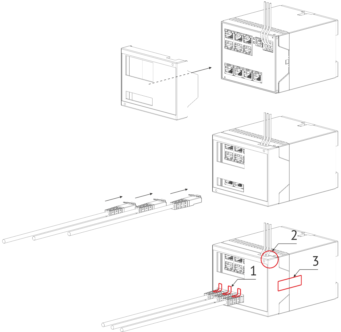
Рисунок Б2. Схема пломбирования устройств ESM-ET и ESM-SV (1 и 3 – место нанесения пломбы-индикатора; 2 – место установки проволоочной пломбы).
