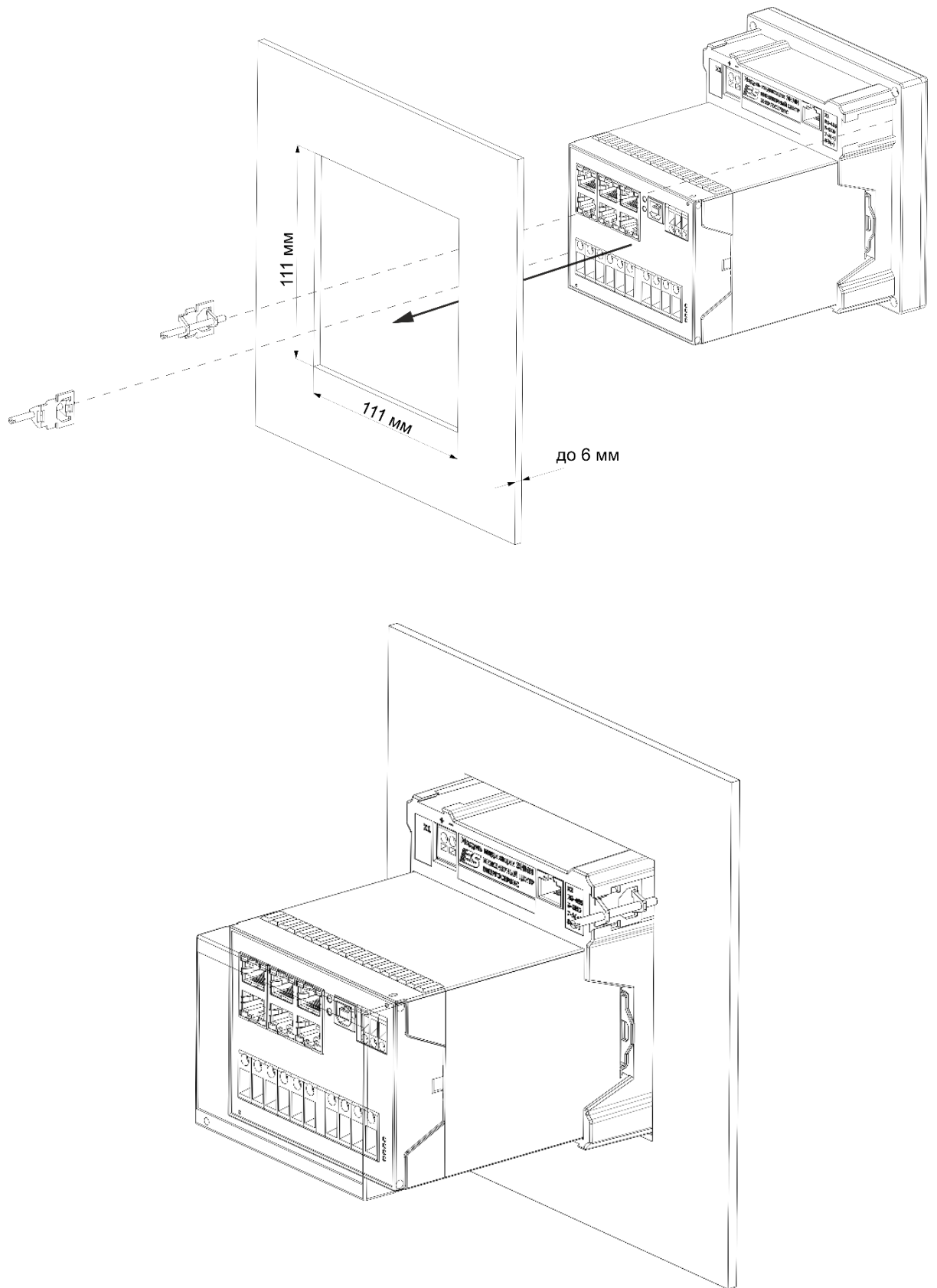
Рисунок 1.7. Схема установки устройства ESM с модулем индикации ЭНМИ-4м в щит
